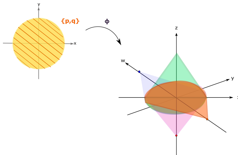
Figura 1.16: Imagen de todos los elementos de la forma \{p, q\} cuando p, q están en cualquier recta paralela a la recta menos identidad.
