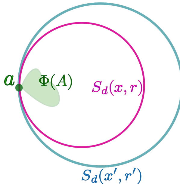
Figura 1.25: Representación en \mathbb{R}^2 de S_d(x, r) , S_d(x', r') y \Phi(A) .
